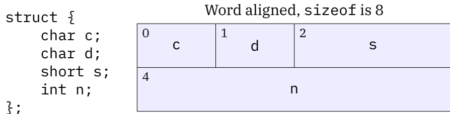
Figure 1.6.: No padding
