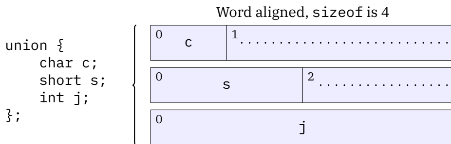
Figure 1.9.: Union padding
