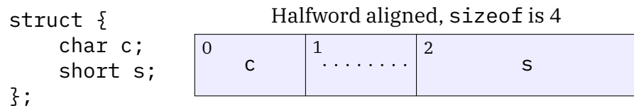
Figure 1.7.: Internal padding
